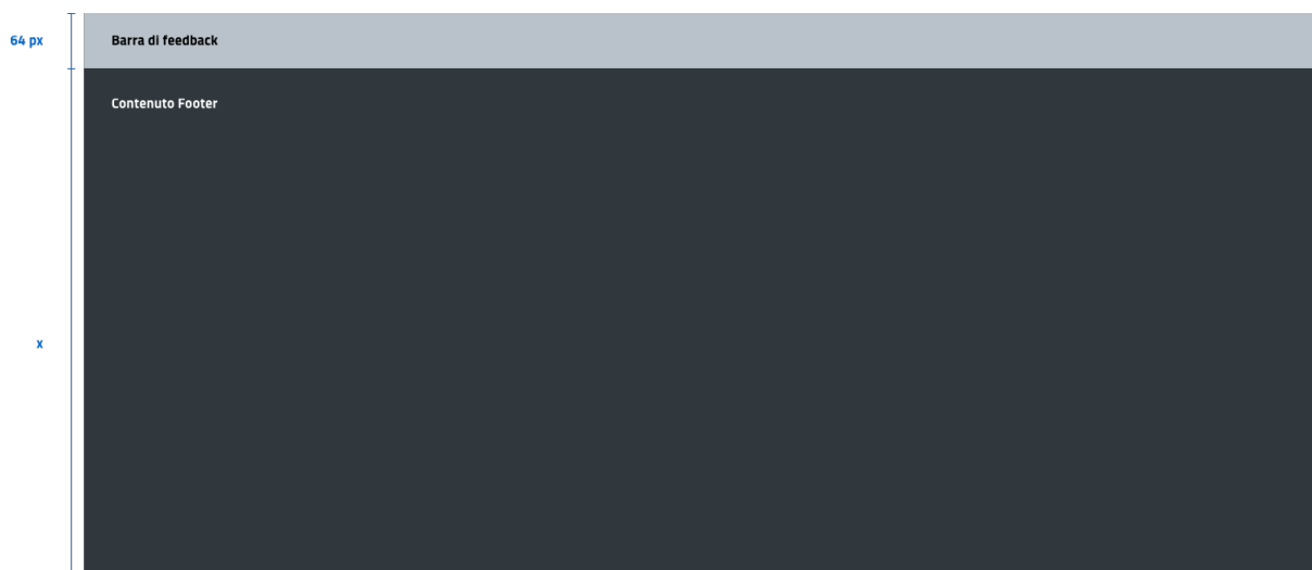
Fig. 5.2: Struttura footer
